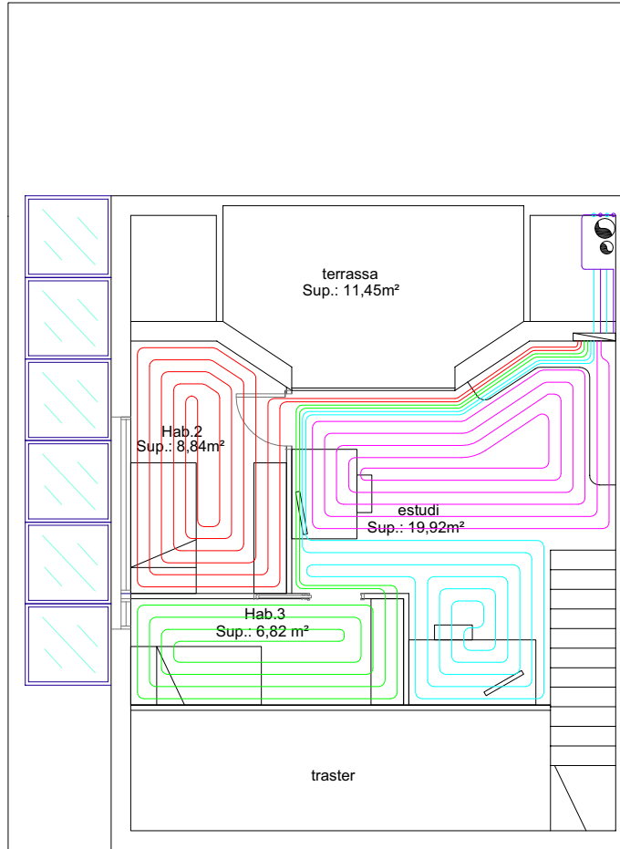
PLANTA SEGONA
