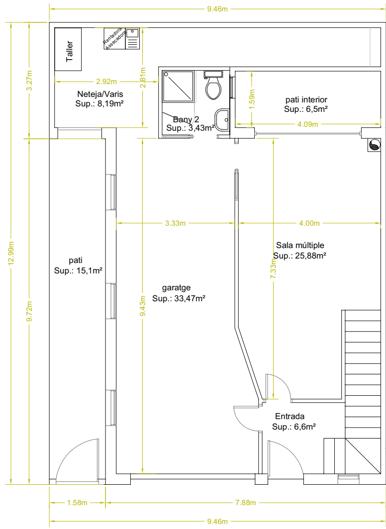
PLANTA BAIXA
