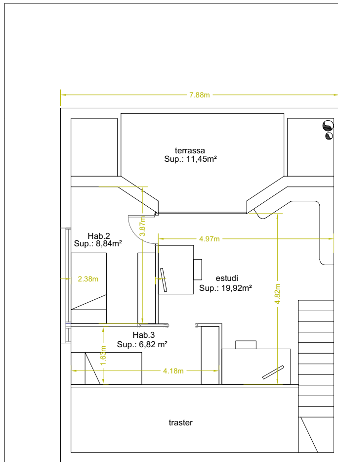
PLANTA SEGONA
