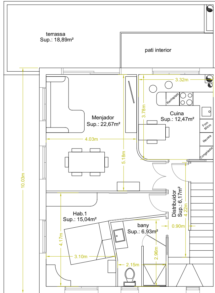
PLANTA PRIMERA
